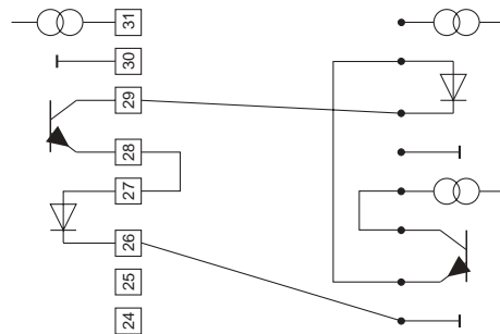
demi-duplex, l'appareil passive
