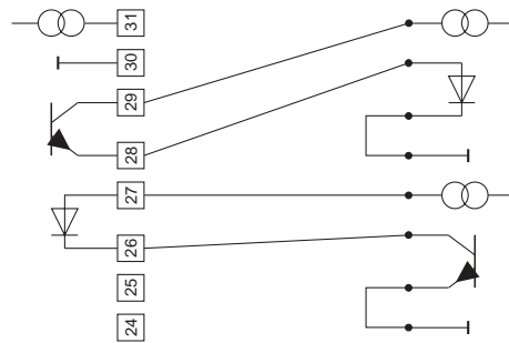
complet-duplex, l'appareil TxD, RxD passive
