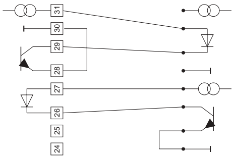
complet-duplex, l'appareil TxD aktive, RxD passive
